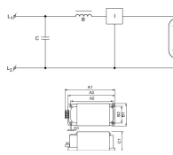
Technische Daten Philips HID-Hochspannung BHD 2000 L76 380 400 415V 50Hz HP-31
